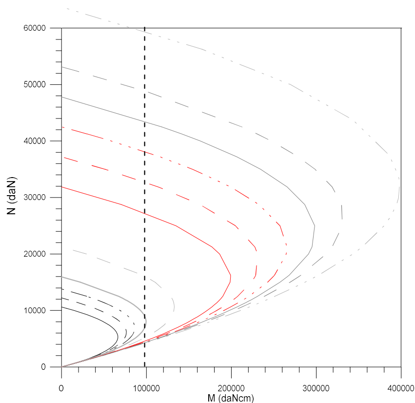
Fig.12. Domini di rottura per diversi valori di resistenza della muratura
