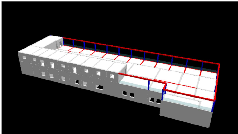
Fig.15. Modello strutturale edificio B6, fronte Est.
