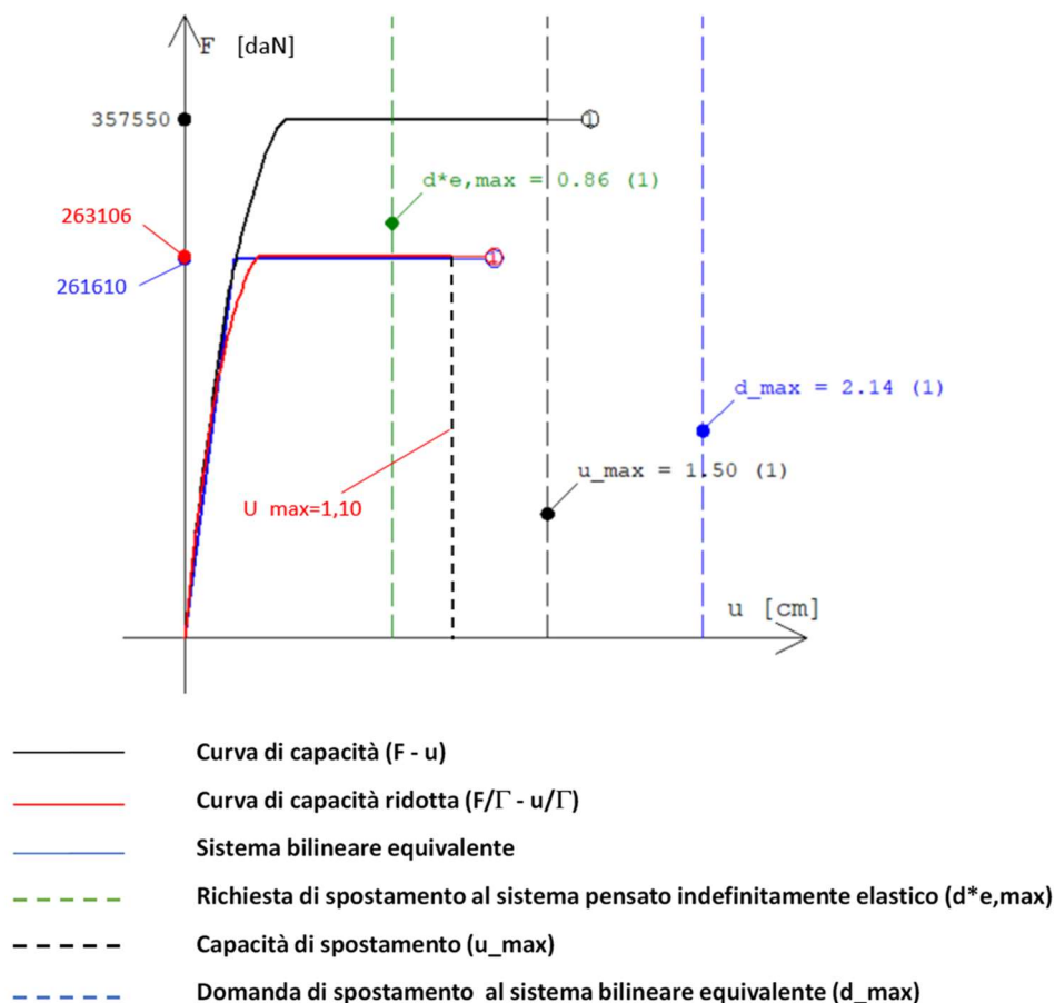
Fig.18. Curve di capacità associate all'indicatore di rischio più basso e confronto con richiesta .
