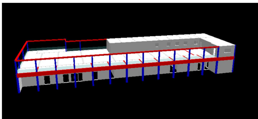
Fig.16. Modello strutturale edificio B6, fronte Ovest.
