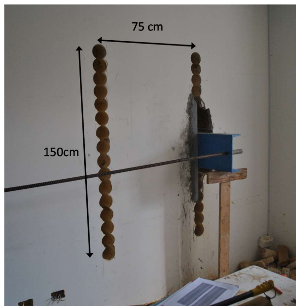
Fig.14. Campione testato a taglio su muro n.2
